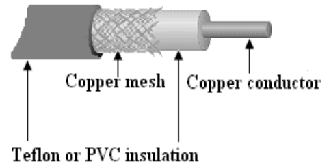
चित्र क. 4.9: कोयेक्सल केबल
