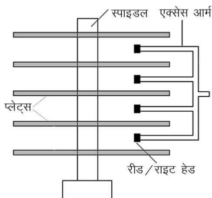
चित्र क. 3.31: हार्ड डिस्क
