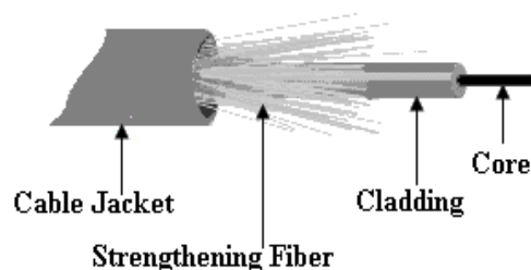
चित्र क. 4.10: फाइबर आप्टिकल केबल
